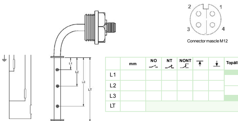
Connexió elèctrica bàsica
