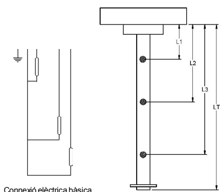
Connexió elèctrica bàsica
